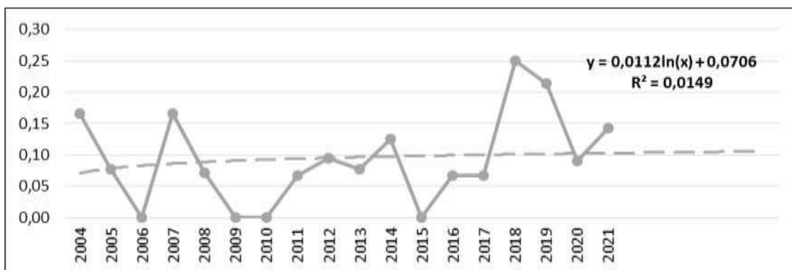
Рис. 3. Зміна метеопотенціалу атмосфери м. Харків у серпні та прогноз до 2026 року
